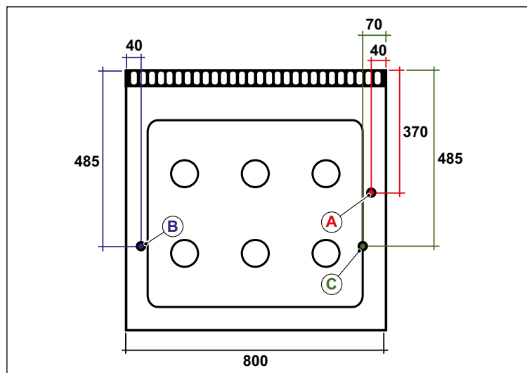
Abb. 12 Wanne 800x700
