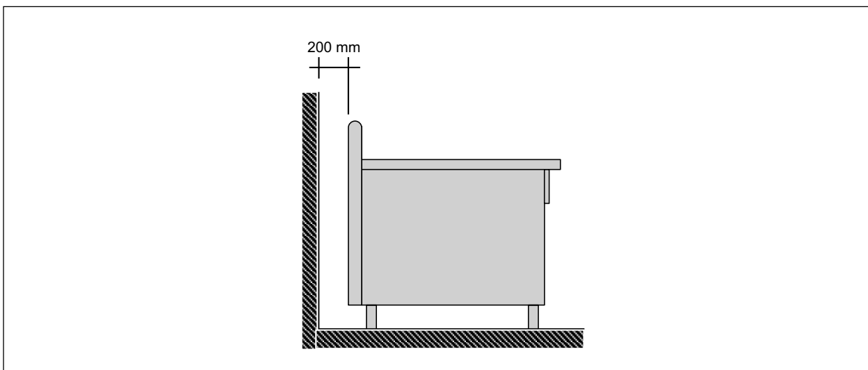
Abb. 13 Minimalabstand von entzündlichen Wänden
