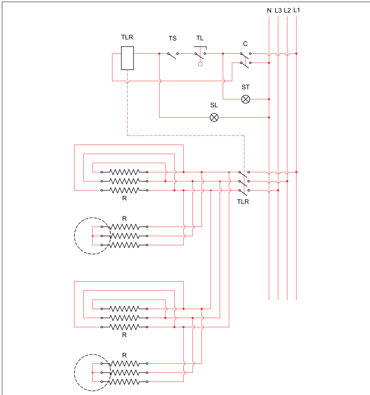
Abb. 17 Stromlaufplan
