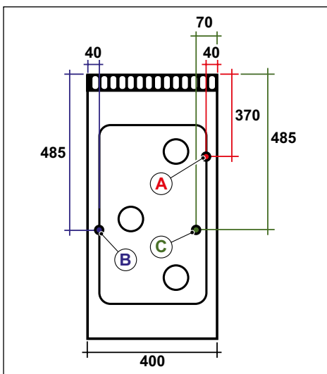
Abb. 11 Wanne 400x700
