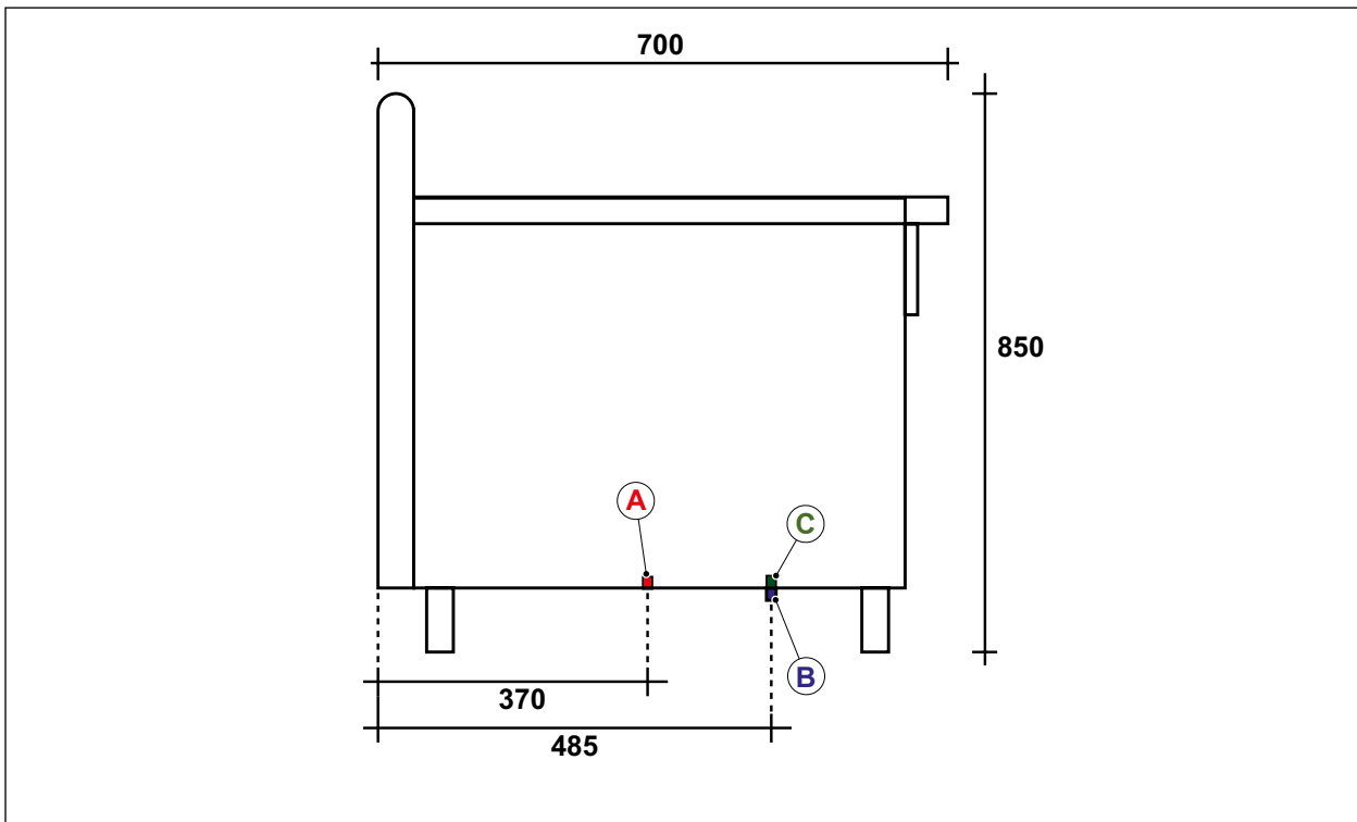
Abb. 10 Abmessungen DIM SUM
