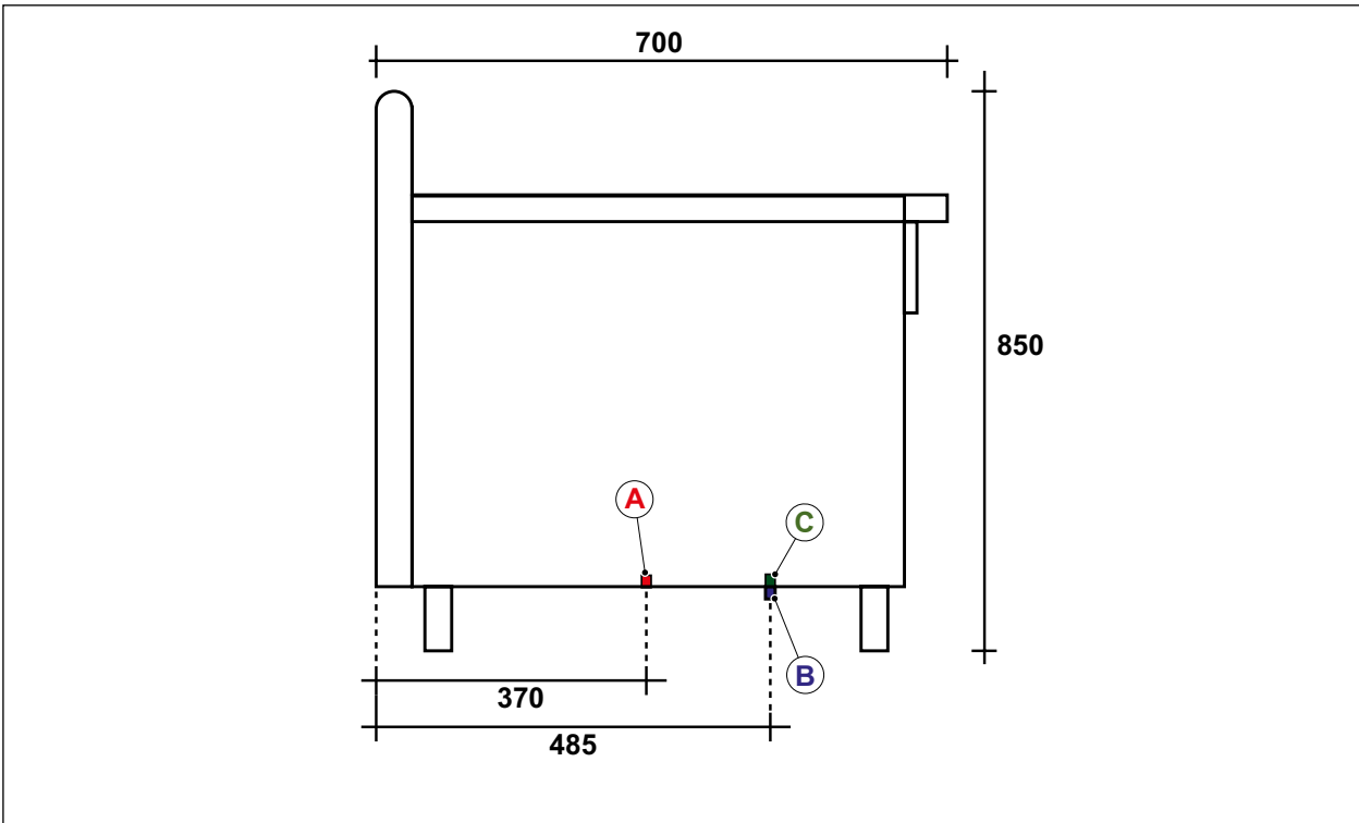
Fig. 10 DIM SUM dimensions
